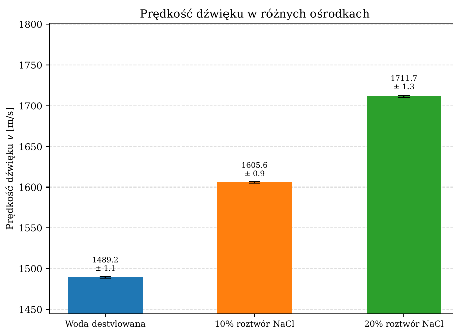
Rysunek 4: Prędkość dźwięku v w badanych ośrodkach. Słupki błędów odpowiadają niepewności u_v wyznaczonej ze wzoru (??).
